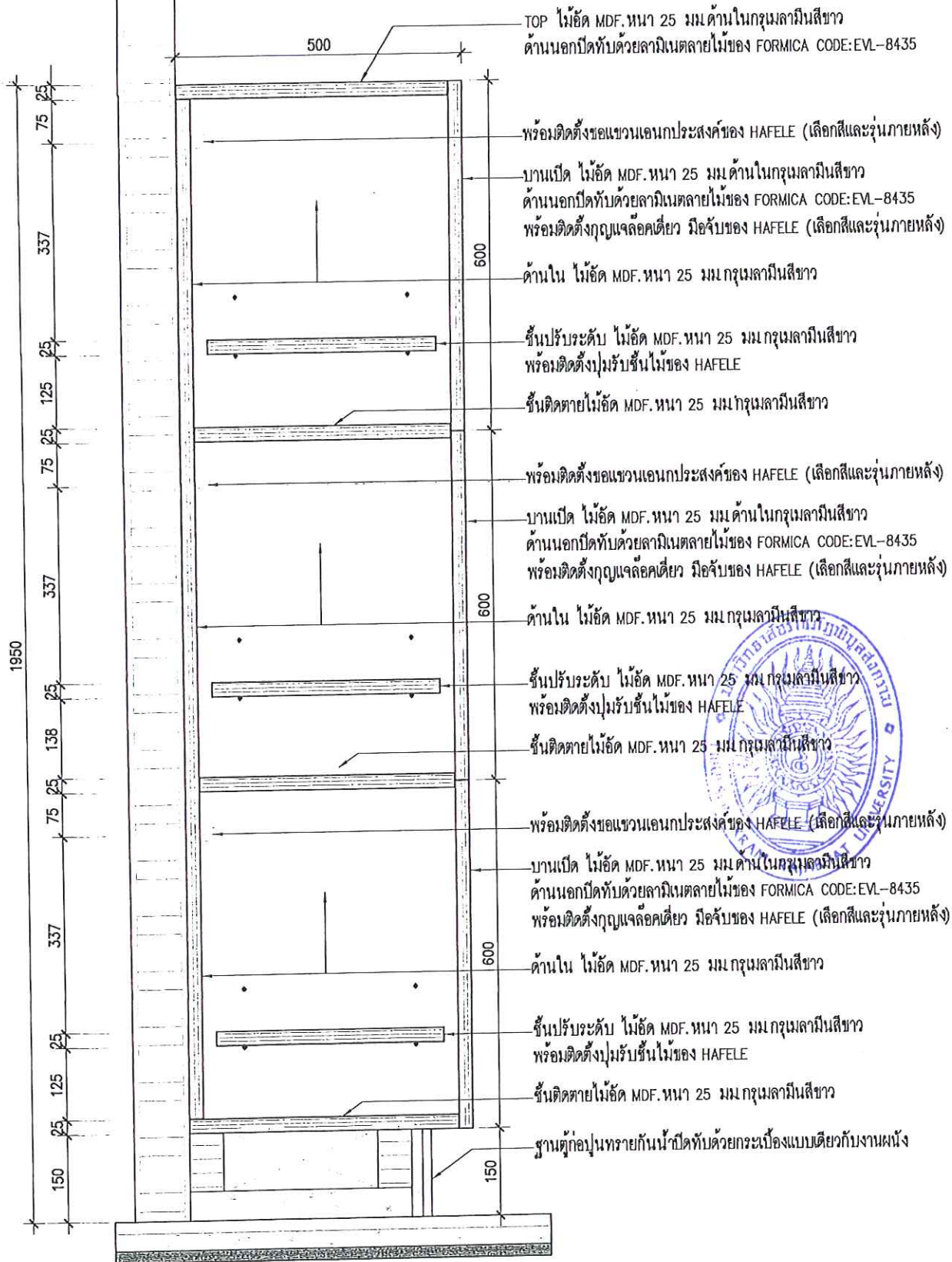
รูปตัด 1 แบบขยาย LOCKER พนักงานชาย SCALE A3 1:10
