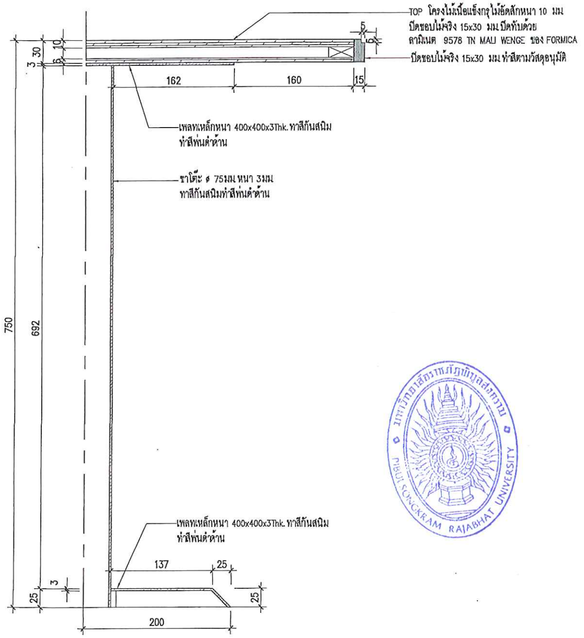
SECTION ๗ โต๊ะทานอาหาร
