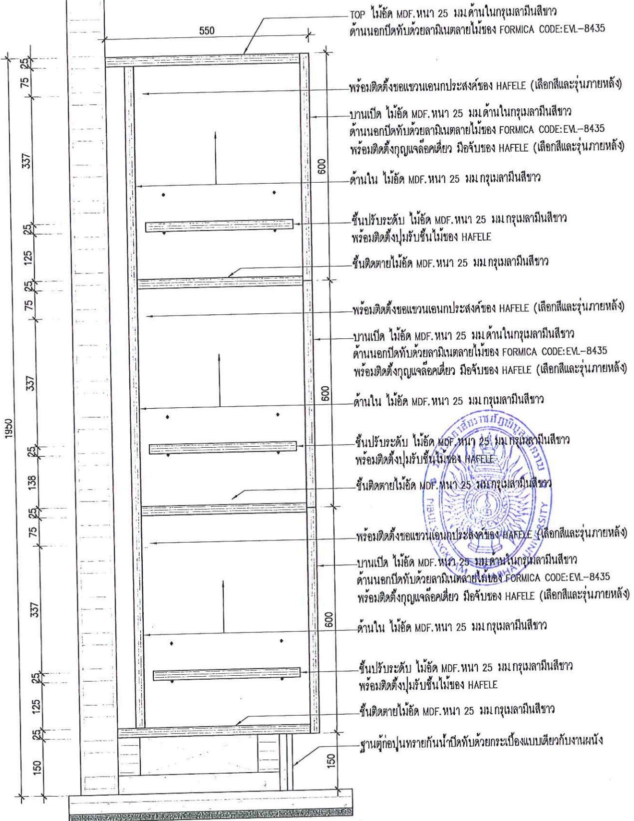
รูปตัด 2 แบบขยาย LOCKER พนักงานชาย SCALE A3 1:10
